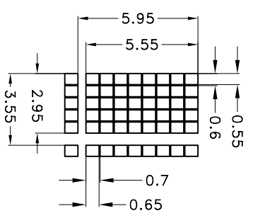
DETAIL DOTS SCALE: 4:1
